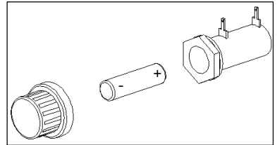
Figura 1 : Montaggio della pila
